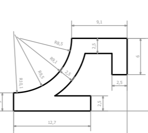
PO_05_007_B_X Mosiądz
