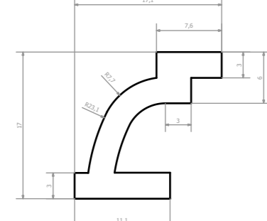
PO_05_002_B_X Mosiądz
